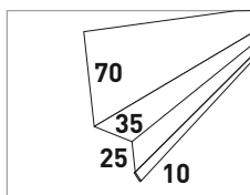
Отлив верхний
