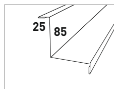
Планка угла внутрен. простая
