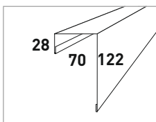
Планка торцевая фасадная
