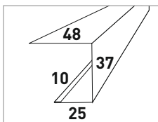
Планка завершающая
