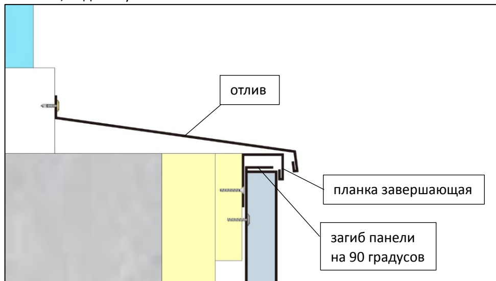
Низ окна, вид сбоку
