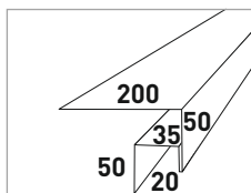
Планка около- оконная сложная
