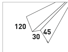
Планка начальная
