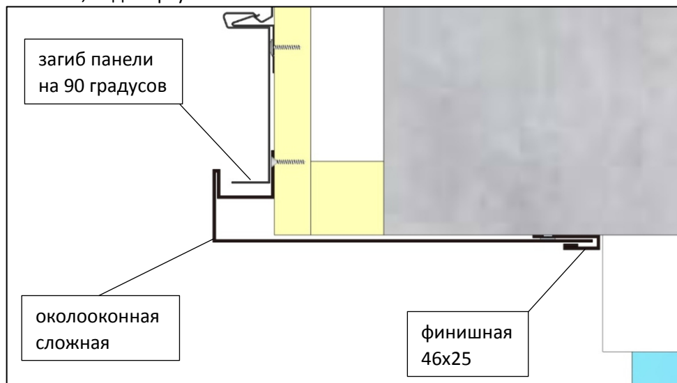
Бок окна, вид сверху
